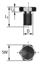
530LF3 Trichterförmiger Schmiernippel M3
