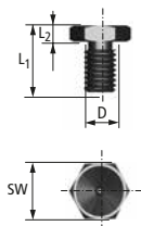
530LF6 Trichterförmiger Schmiernippel M6
