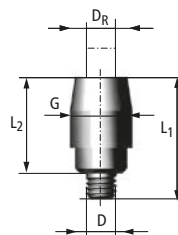
530LA3 Gerader Einschraubanschluss M3 Für Leitungen mit Außendurchmesser D R = 3 mm
