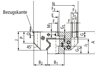
512 Ausführung A
