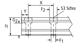
512 Ausführung B
